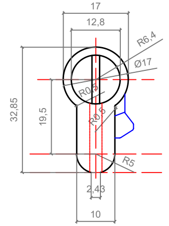
A-A KESİTİ
