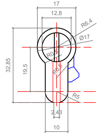
A-A KESİTİ
