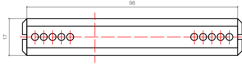
ALT GÖRÜNÜŞ
