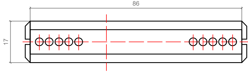
ALT GÖRÜNÜŞ
