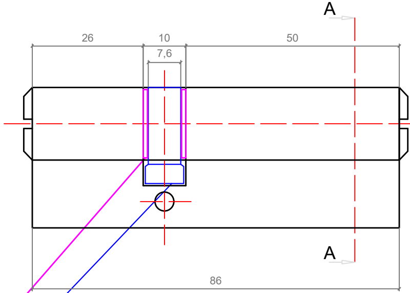
ALT GÖRÜNÜŞ
