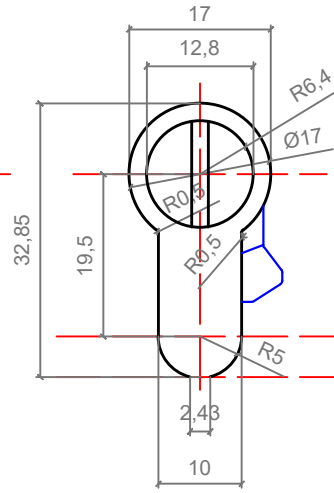
GÖRÜNÜŞ
