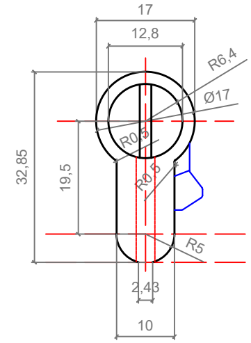
A-A KESİTİ
