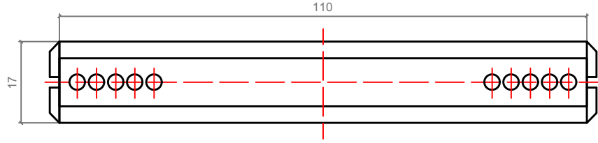
ALT GÖRÜNÜŞ
