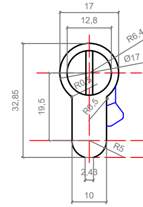
GÖRÜNÜŞ
