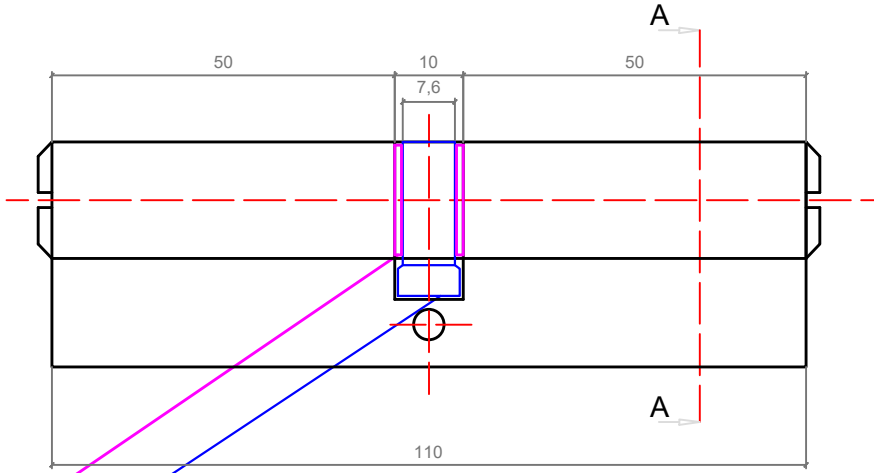
ALT GÖRÜNÜŞ
