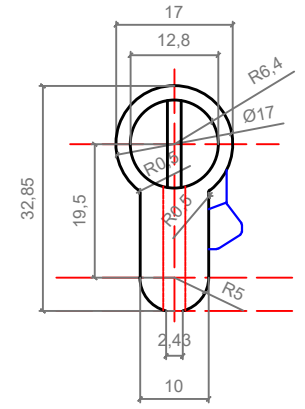
A-A KESİTİ
