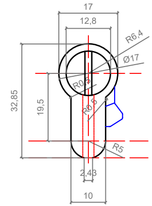
A-A KESİTİ
