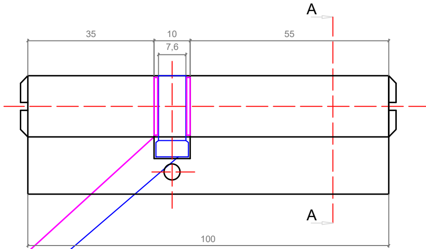
ALT GÖRÜNÜŞ
