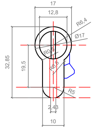
A-A KESİTİ
