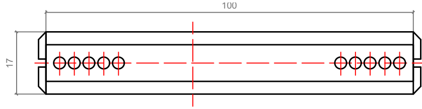
ALT GÖRÜNÜŞ
